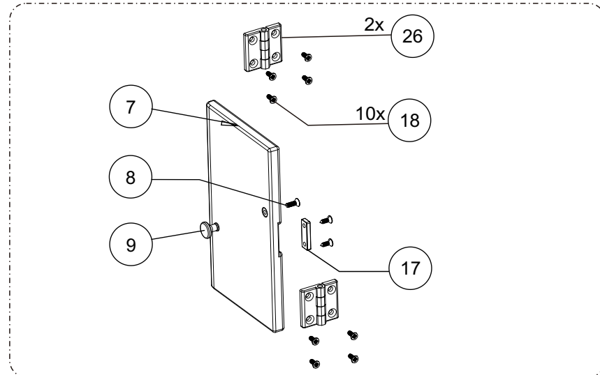
Door Assm Unit
