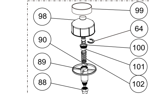
Air Vortex Cap Assm
